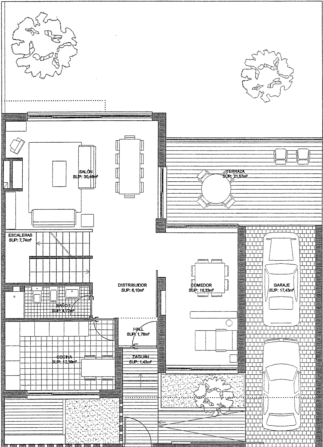
PLANTA BAJA
