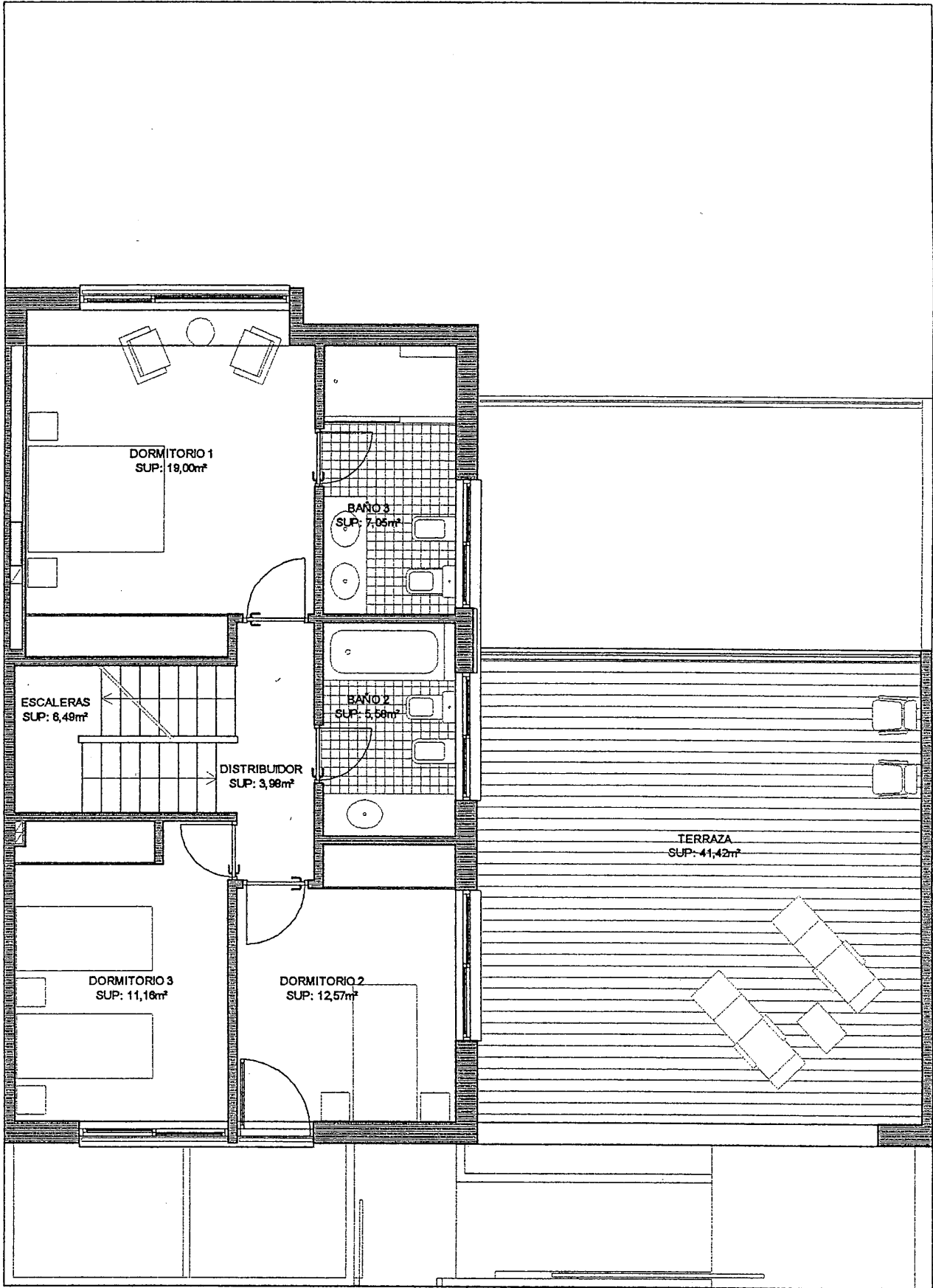
PLANTA PRIMERA
